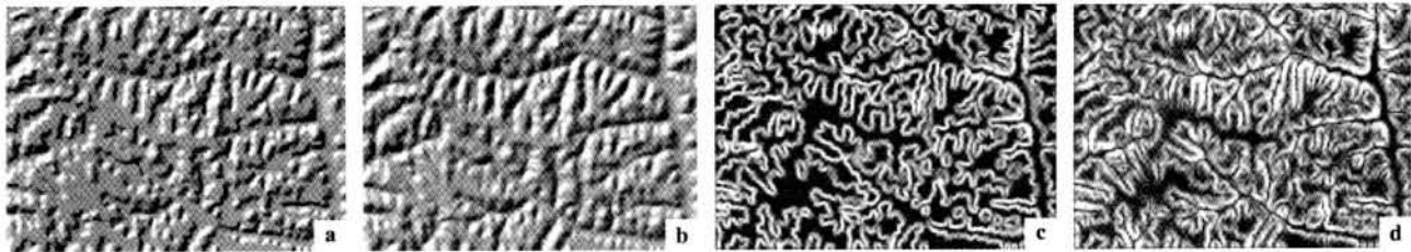
图 1 不同类型 DEM 生成的光照模拟和和提取的坡度
