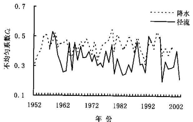
图2 延河流域降水、径流不均匀系数
