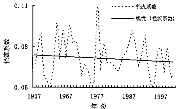
图 4 流域径流系数变化过程
