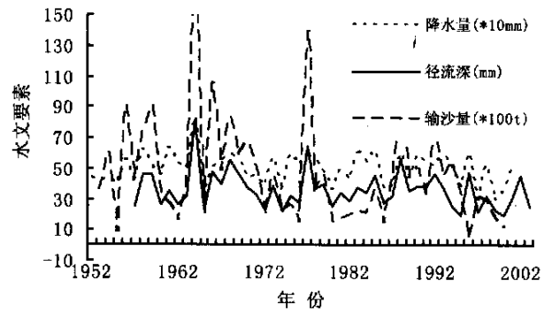
图 3 延河流域水文要素时变过程
