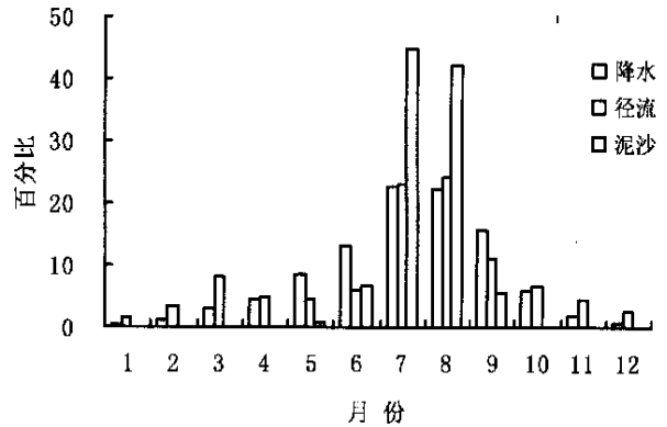
图1 延河流域水文要素分配
